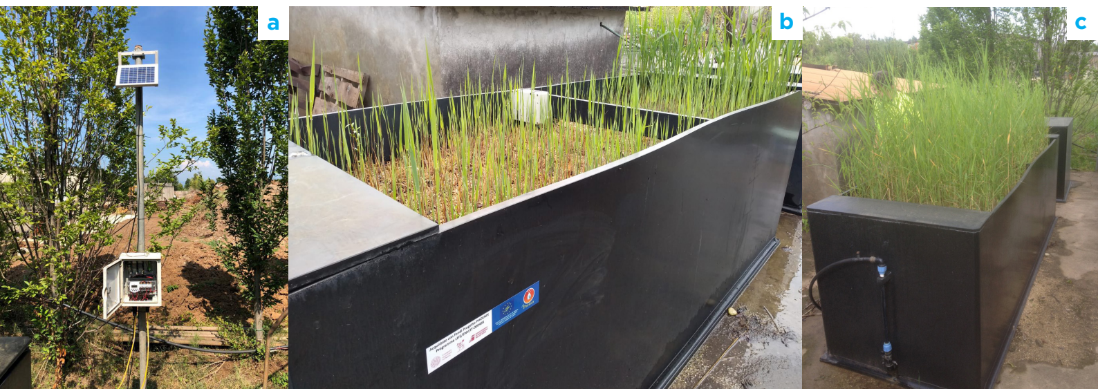
Centralina di controllo delle pompe per l'afflusso di acqua (a). La centralina è alimentata da energia solare (vedi il pannello in alto a sx). Phragmites australis , primavera 2018: b) in aprile, c) in maggio.
