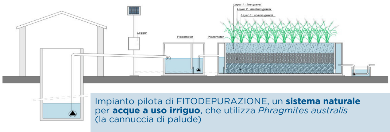
Impianto pilota (3 m 3 ) riempito con acqua contaminata, per valutare la capacità di assorbimento delle piante nel rimuovere i PFAS.
